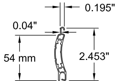
1 SLAT 6063-T6
