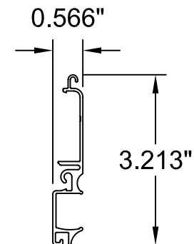
7 BOTTOM SLAT
